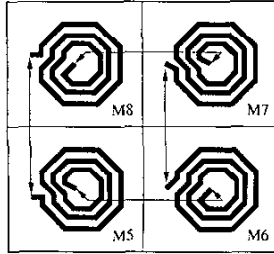
Fig. 7. MTS inductor diagram
