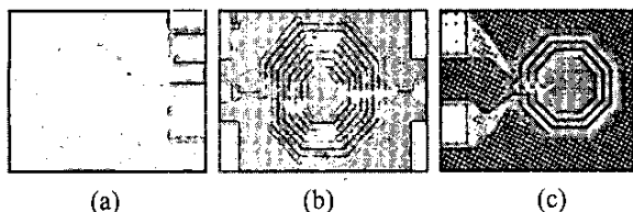
Fig. 11. Microphotographs for on-chip inductors ((a). STP(4) inductor (b). MTP7.5T2 inductor (c). MTS3T8 inductor)
